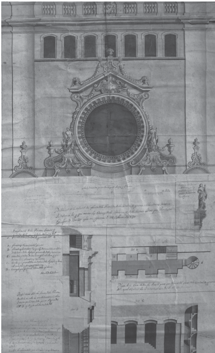
Figura 9. Traça parcial de la façana de la catedral de Girona, que guiaria les obres d'acabament del frontis (1730). Tinta i aiguada sobre paper (90 cm d'alt x 40 cm d'ample). Arxiu Capítular de Girona. Fotografia: FM-ACG.
